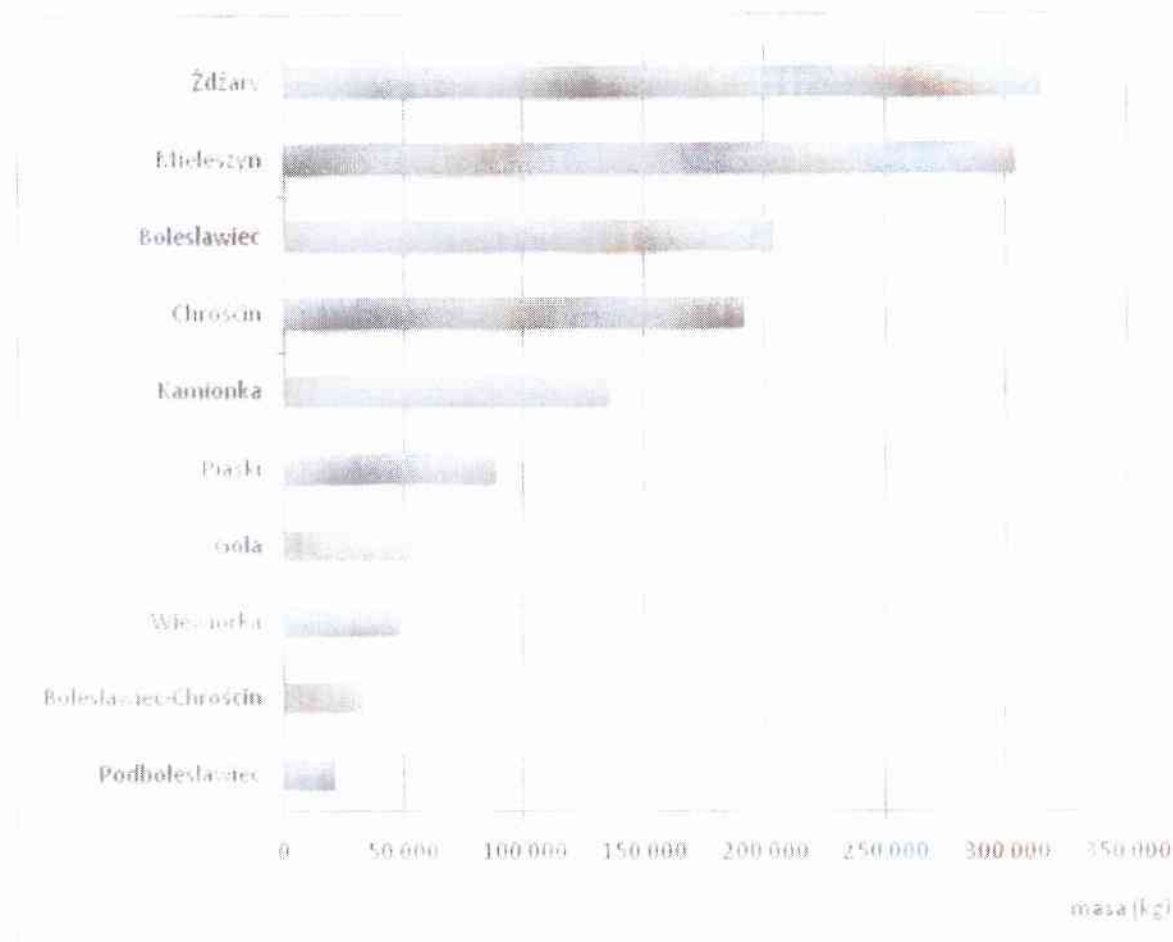
Rys. 5. Porównanie ilości zinwentaryzowanych wyrobów zawierających azbest dla poszczególnych obrębów ewidencyjnych Gminy Bolesławiec (kg).
